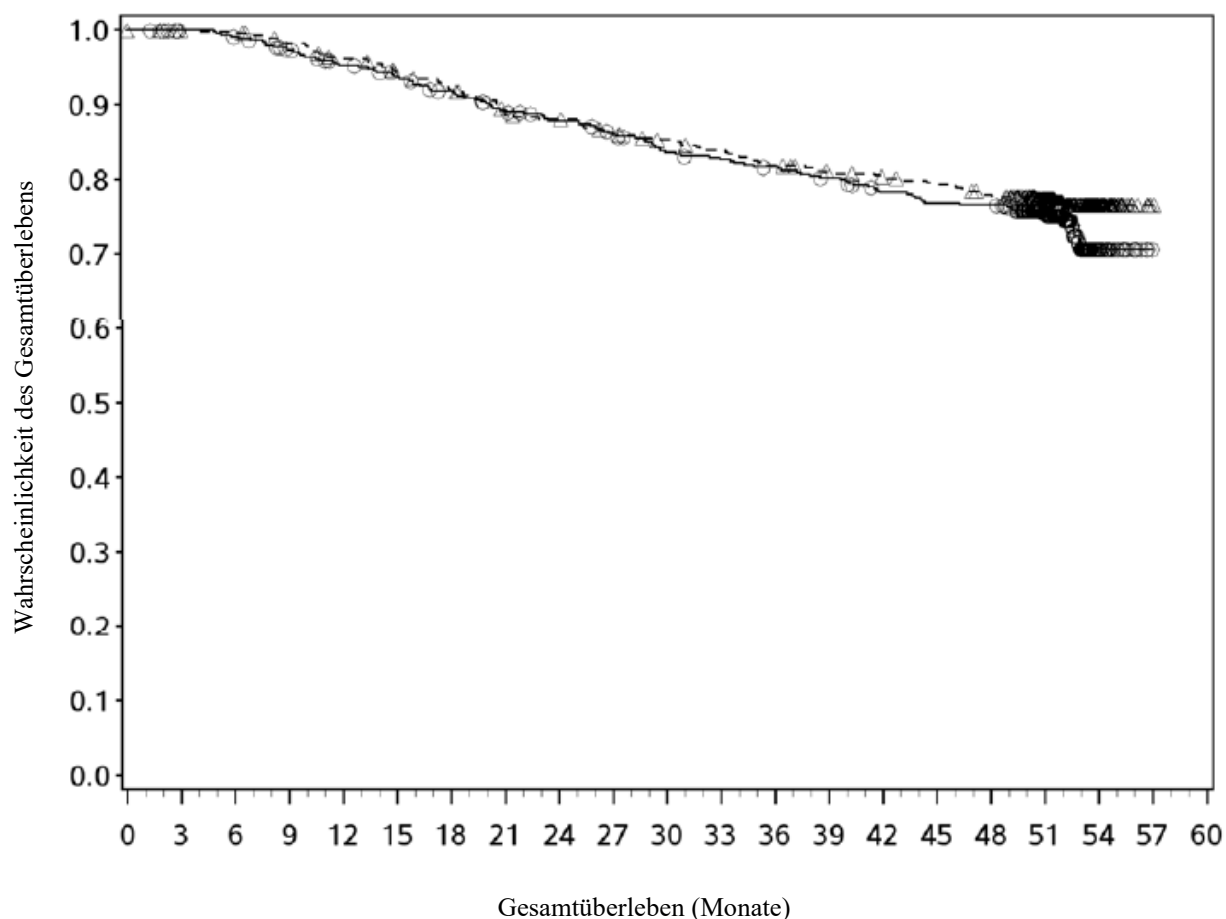
Abbildung 3: Gesamtüberleben (CA209238)
